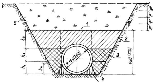
Рис. 4. Схема уплотнения грунта при засыпке траншеи:
