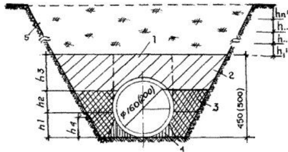
Рис. 1. Схема уплотнения грунта при засыпке траншей:
