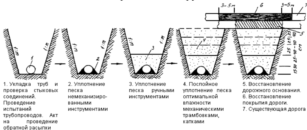
Рис.2. Последовательность работ по восстановлению дорожной конструкции
